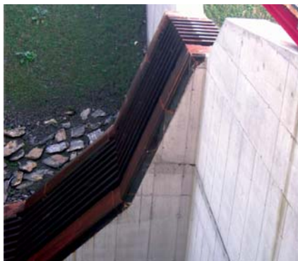
3. ábra: Iszapfogó
