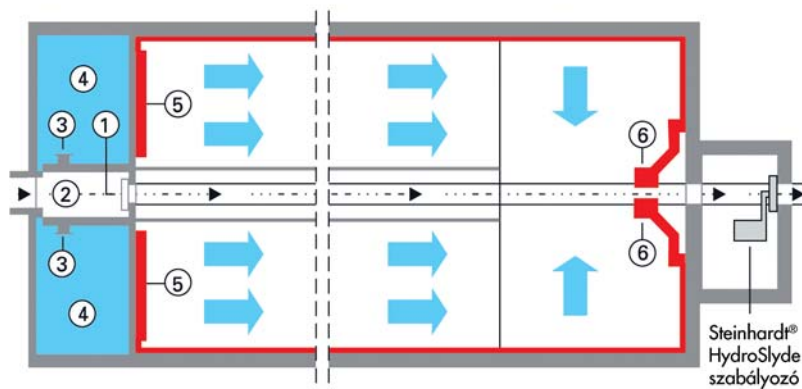
A HydroSelf csatornahullám öblítőcsappantyú működése egy átfolyós tározóban
