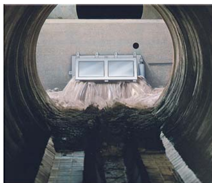
HydroSelf csatornahullám öblítőcsappantyú csatornatározóba építve
